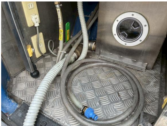
排水タンク（200ℓ） 給排水口 直結ホース
