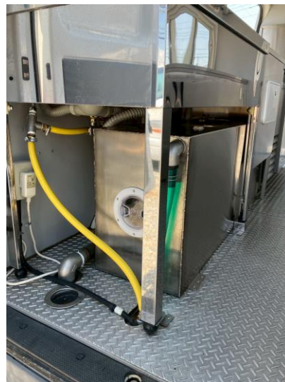
給排水タンク (200ℓ)
